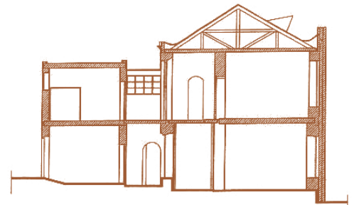
↑ برش ج - ج: بخشی از مدرسه دارالفنون
