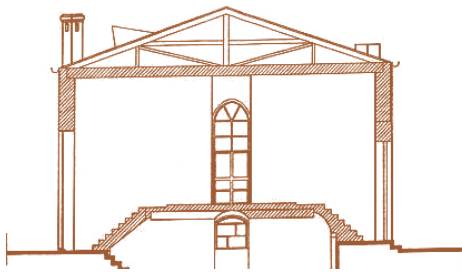
↑ برش ه - ه: بخشی از مدرسه دارالفنون
