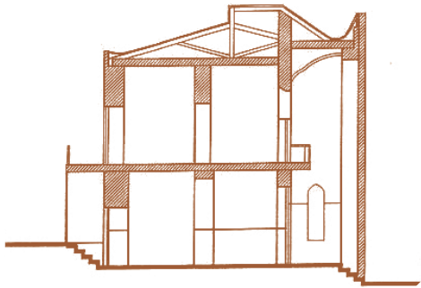
↑ برش ب - ب: بخشی از مدرسه دارالفنون
